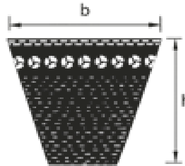
Profil XPA h: 10,0 mm · b: 12,7 mm · m: 0,105 kg/m
