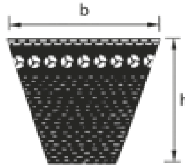
Profil XPZ h: 8,0 mm · b: 9,7 mm · m: 0,065 kg/m
