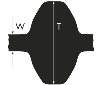
Profil DS8M h_s: 7,50 \text{ mm} \cdot t: 8,00 \text{ mm}
