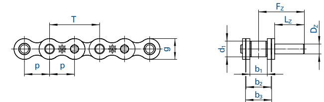
Form F Einseitige Mitnehmerbolzen (auch versetzt wechselseitig möglich)
