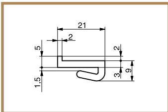
Klemm-L-Profil 21 x 11
