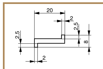
Z-Profil 20 x 8
