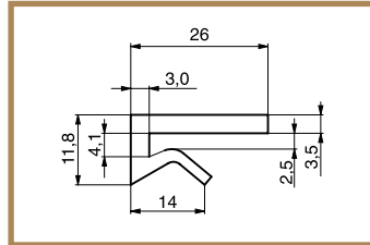
Klemm-Flach-Profil 26 x 11,8
