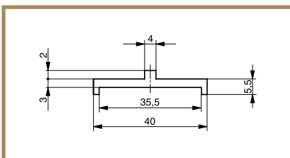
Steg-Wulst-Profil 40 x 7,5
