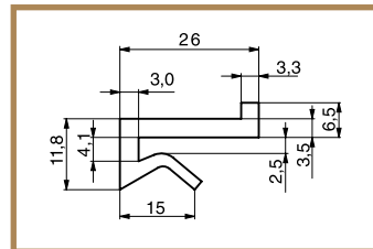
Klemm-L-Profil 26 x 14,8
