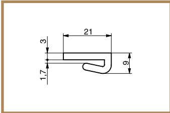
Klemm-Flach-Profil 21 x 9
