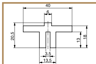
T-Aufsteck-Profil 40 x 20,5
