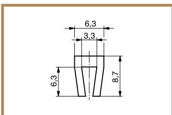
Klemm-U-Profil 6,3 x 8,7
