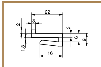
Klemm-L-Profil 22 x 11
