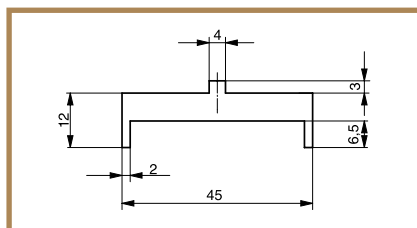
Steg-Wulst-Profil 45 x 15
