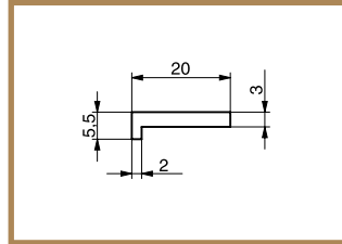
L-Profil 20 x 5,5
